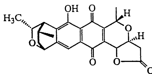
GRANATICIN (4)
