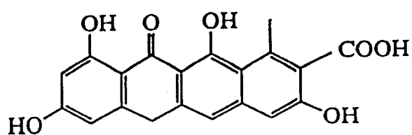
TETRACENOMYCIN F1 (5)
