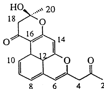
RM 20 (9)
