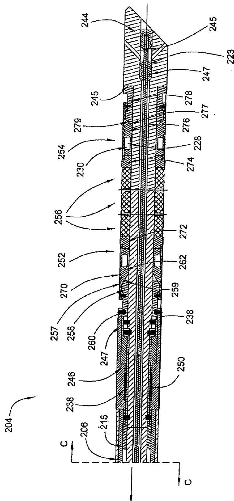
FIG. 3C
