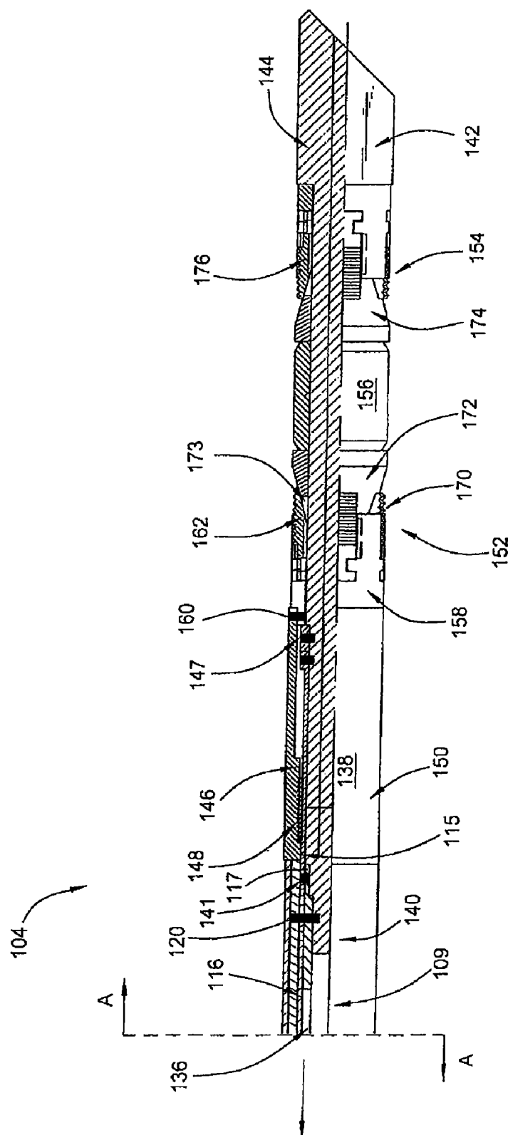
FIG. 1C
