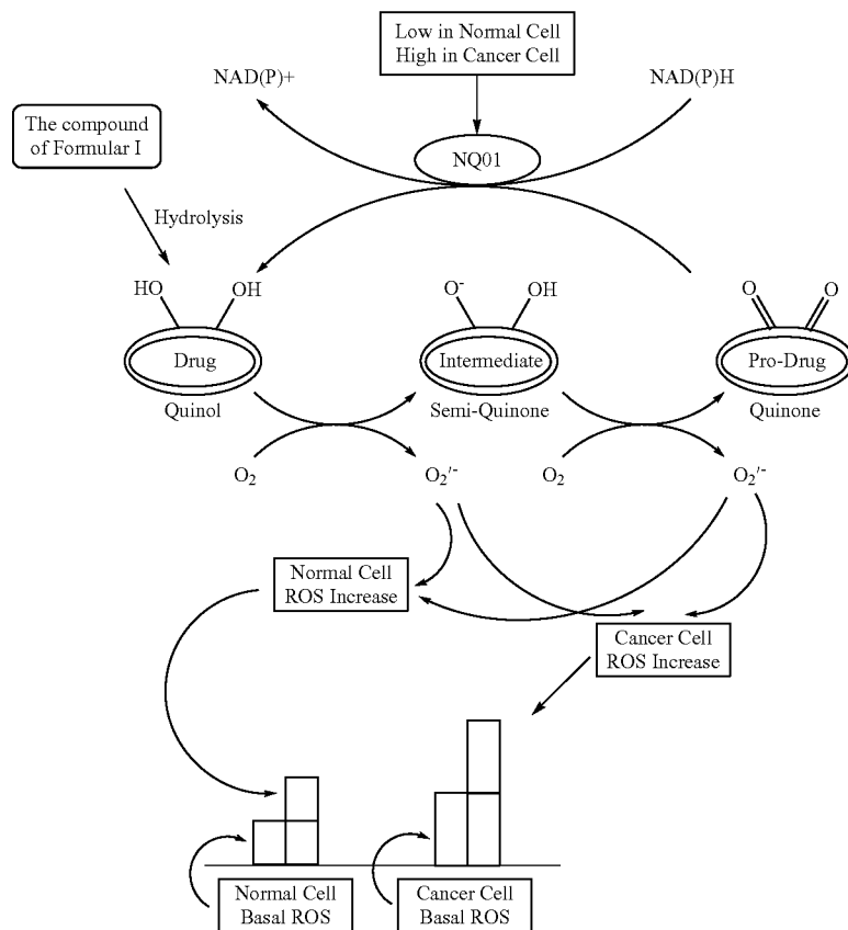
Scheme VIII:
