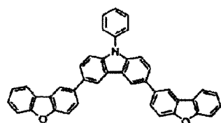
化合物 (H 1)
