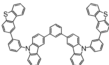
化合物 (H 5)
