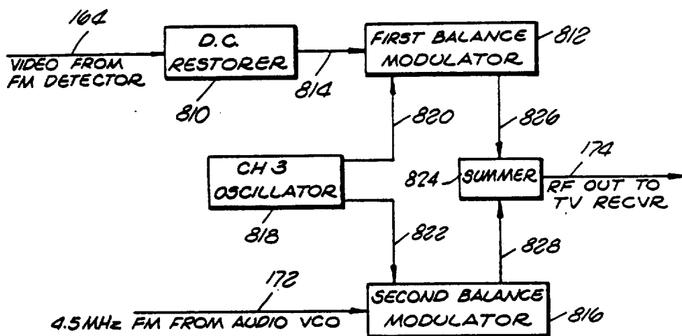
FIG. 24 RF MODULATOR
