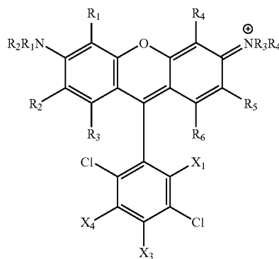
4,7-Dichlororhodamine
