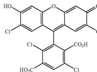
TET
