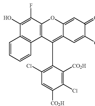
Cl-FLAN
