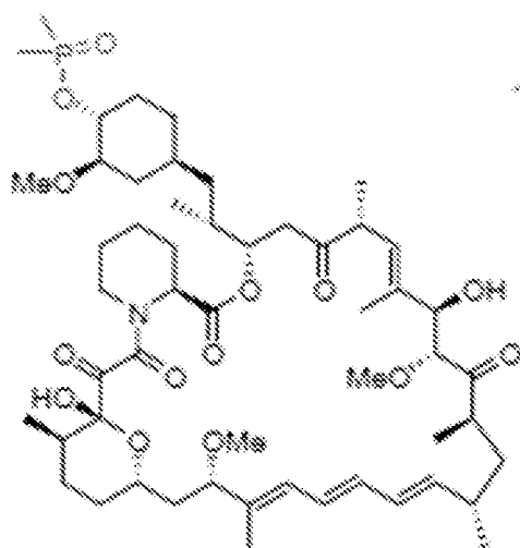
Ridaforolimus (MK-8669)
