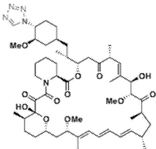
Zotarolimus (ABT-578)
