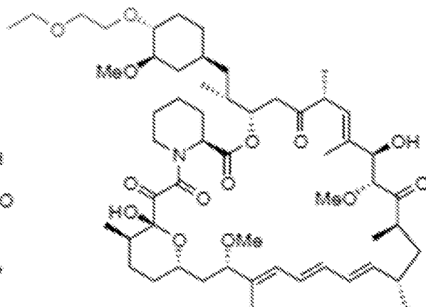
Umirolimus
