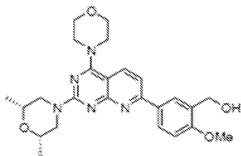
KU-0063794
