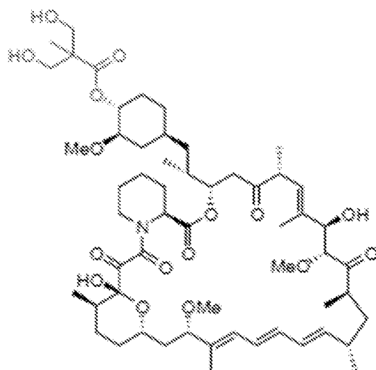
Temsirolimus (CCI-779)
