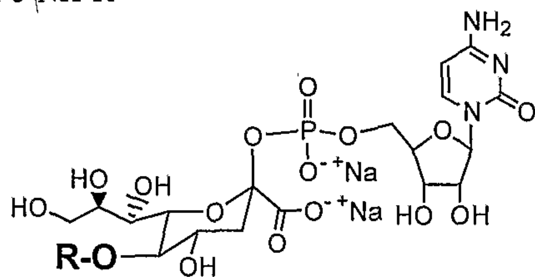
CMP-SA-5-NH-R
