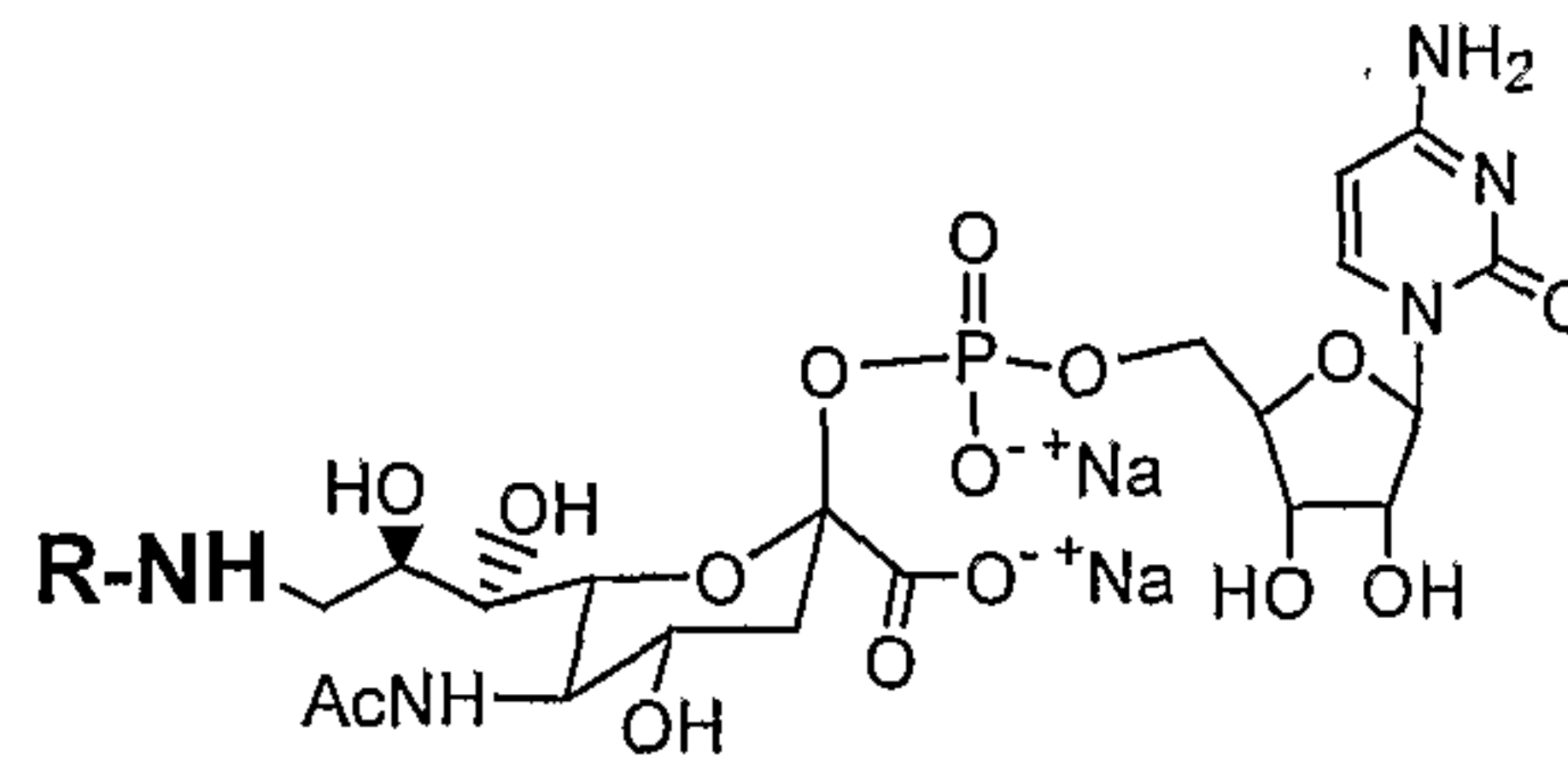
CMP-NeuAc-9-NH-R
