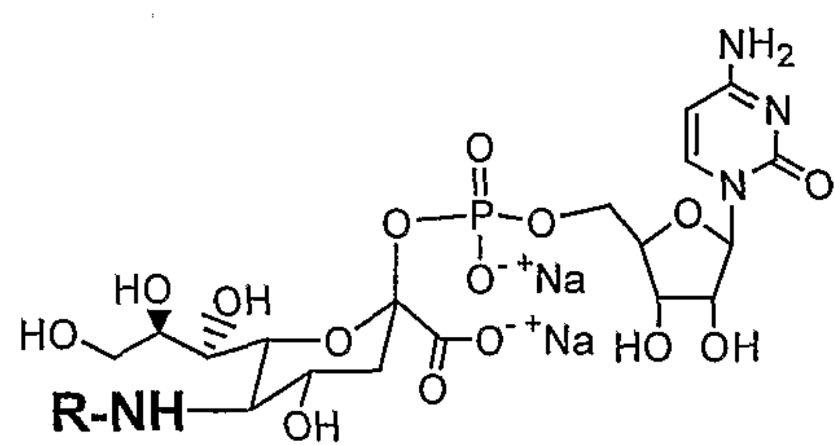
CMP-SA-5-NH-R
