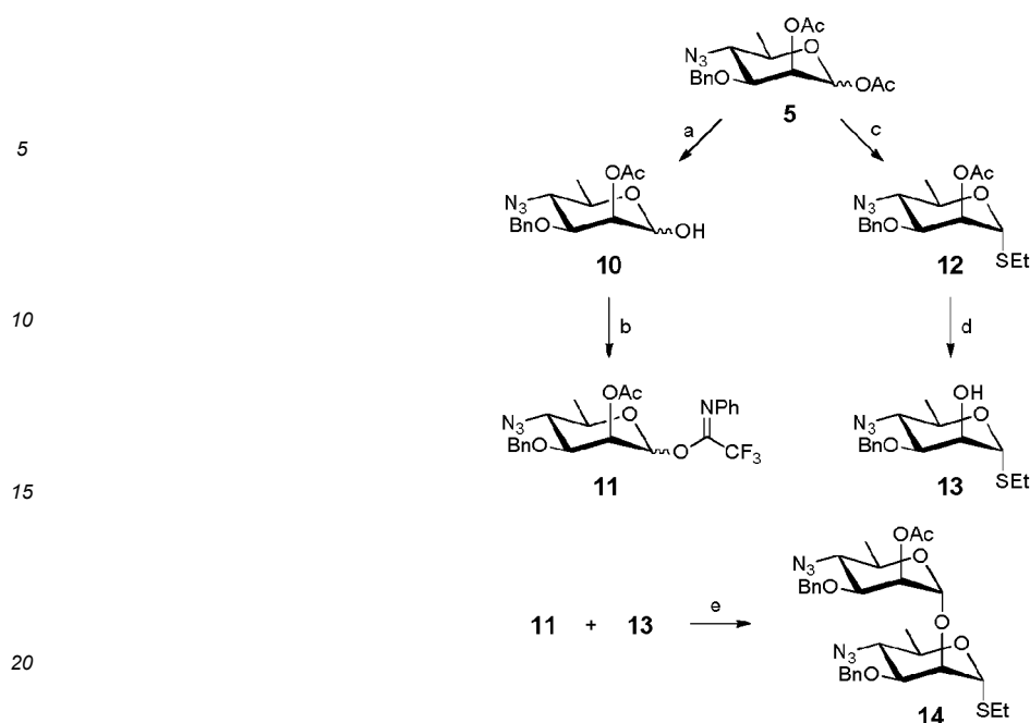
Scheme 2. a) 2M Me 2 NH/THF, CH 2 Cl 2 ; b) CF 3 C(NPh)Cl, Cs 2 CO 3 , CH 2 Cl 2 ; c) EtSH, BF 3 •Et 2 O, CH 2 Cl 2 ; d) NaOCH 3 , CH 3 OH; e) TMSOTf, CH 2 Cl 2 .
