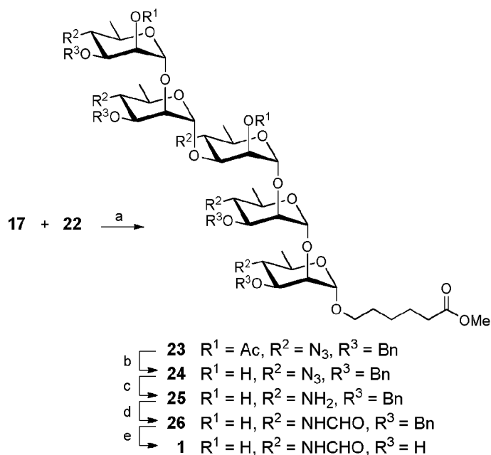
Scheme 5. a) TMSOTf, CH 2 Cl 2 ; b) NaOCH 3 , CH 3 OH; c) H 2 S, Py./NEt 3 1:1; d) Ac 2 O/HCOOH 2:1, CH 3 OH; e) H 2 , Pd/C, AcOH.
