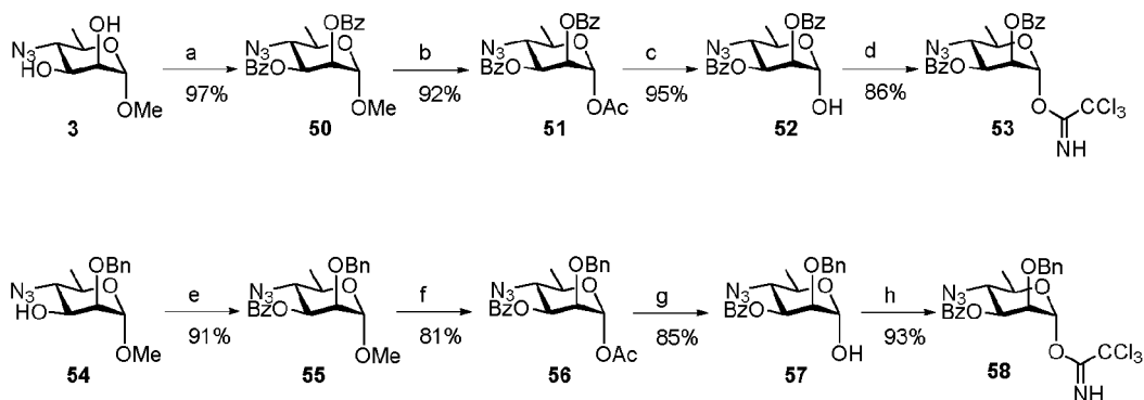
Scheme 9. a) BzCl, Py, rt, 10 h; b) Ac 2 O, AcOH, H 2 SO 4 , rt, 6 h; c) NH 2 NH 2 ·AcOH, DMF, 60 °C, 0.5 h; d) CCl 3 CN, DBU, CH 2 Cl 2 , rt, 10 min.; e) BzCl, Py, rt, 3 h; f) Ac 2 O, AcOH, H 2 SO 4 , rt, 3 h; g) NH 2 NH 2 ·AcOH, DMF, 60 °C, 0.5 h; h) CCl 3 CN, DBU, CH 2 Cl 2 , rt, 10 min.
