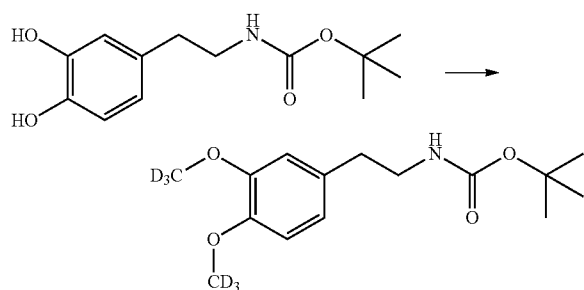
D 6 -tert-butyl 3,4-dimethoxyphenethylcarbamate
