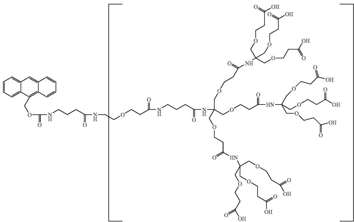
A-[27]-acid:
