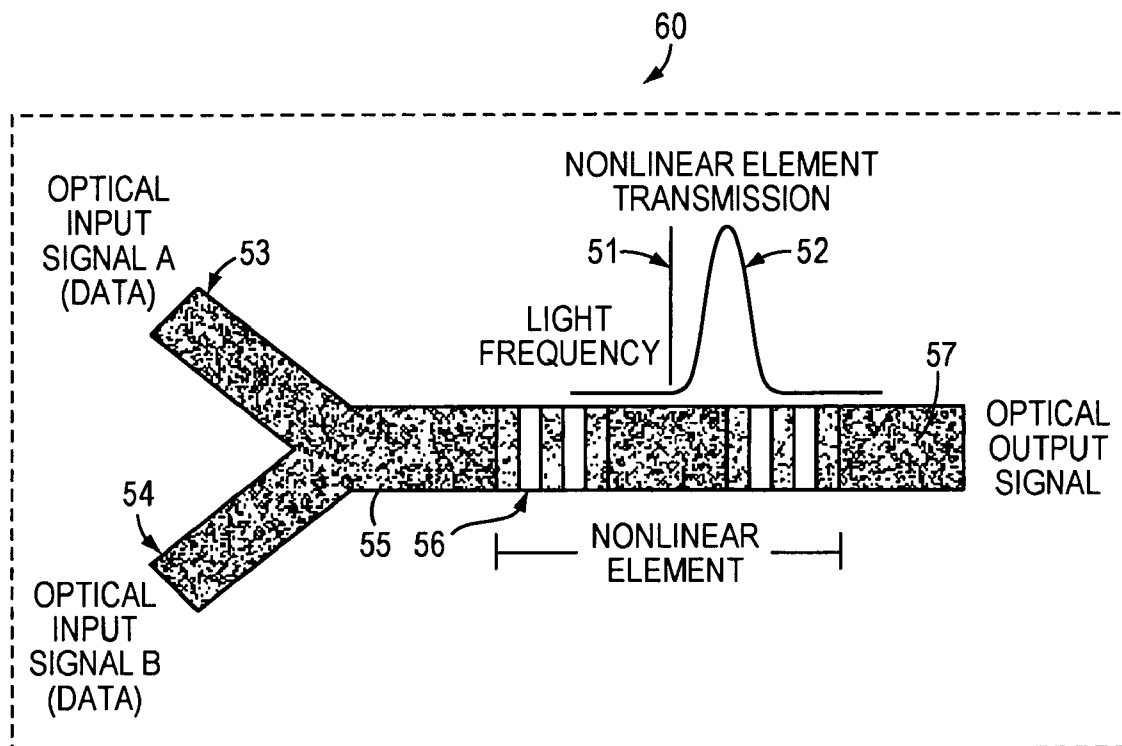
ALL-OPTICAL XOR GATE
