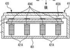
(B) H-H断面図
