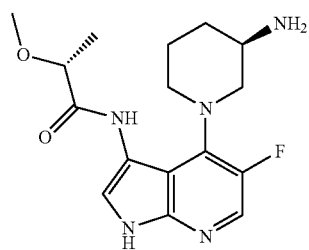
(R)-N-(4-((R)-3-Aminopiperidin-1-yl)-5-fluoro-1H-pyrrolo[2,3-b]pyridin-3-yl)-2-methoxypropanamide
