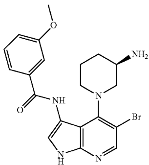
(R)-N-(4-(3-Aminopiperidin-1-yl)-5-bromo-1H-pyrrolo[2,3-b]pyridin-3-yl)-3-methoxybenzamide
