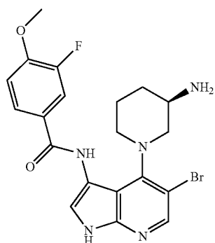
(R)-N-(4-(3-Aminopiperidin-1-yl)-5-bromo-1H-pyrrolo[2,3-b]pyridin-3-yl)-3-fluoro-4-methoxybenzamide
