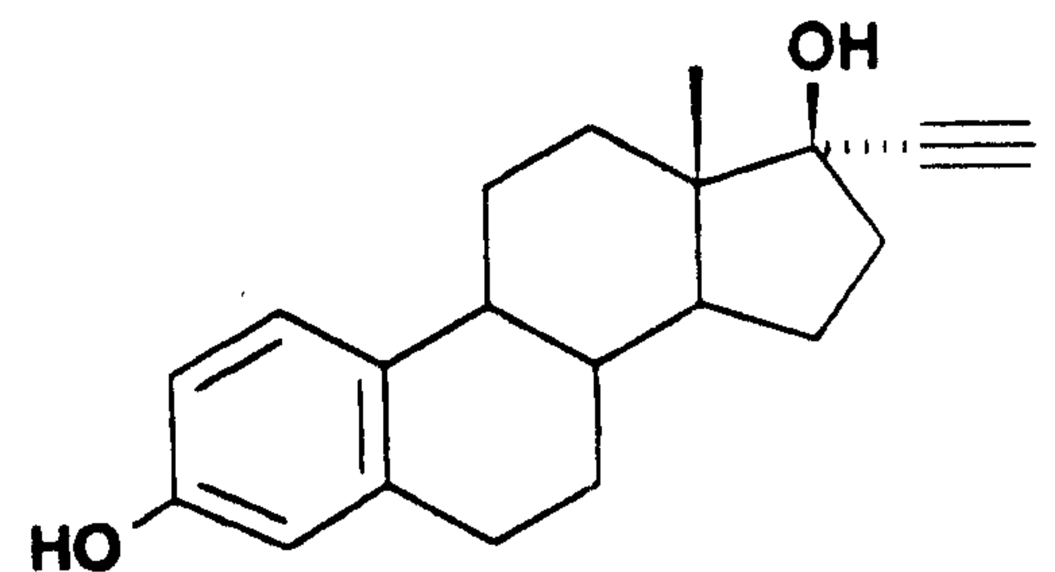
17 \alpha -ETHYNYL-1,3,5(10)-ESTRATRIEN- 3,17 \beta -DIOL
