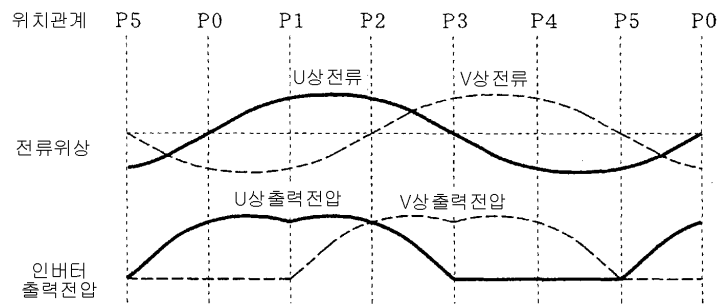
(b) 전 계자의 상태
