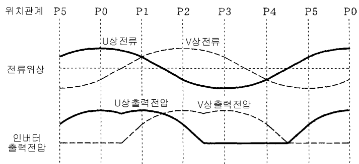
(c) 약 계자의 상태
