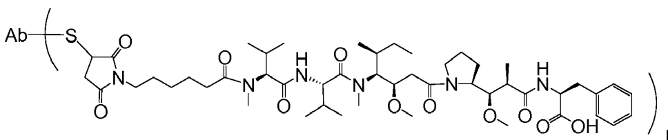
Ab-MC-MMAF
