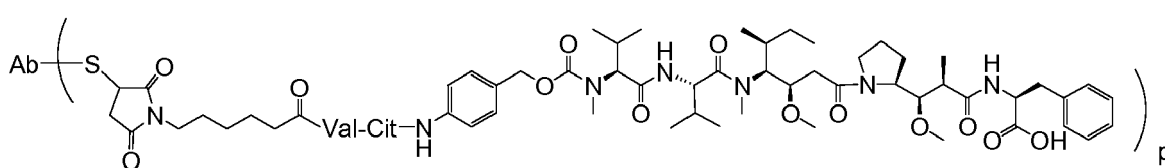
Ab-MC-vc-PAB-MMAF
