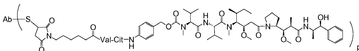
Ab-MC-vc-PAB-MMAE
