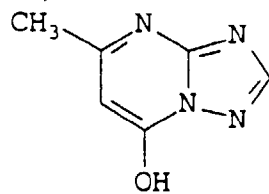
(Cpd - 21)
