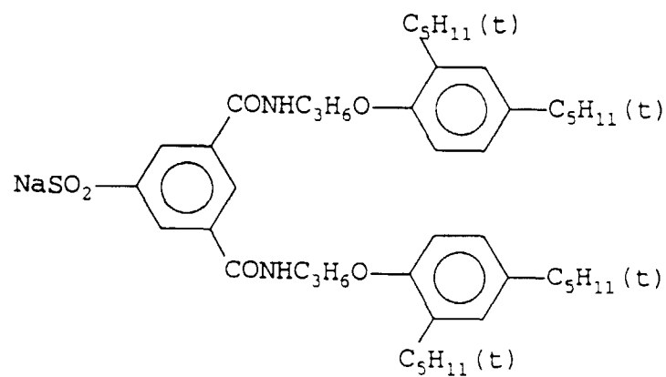
(Cpd - 10)
