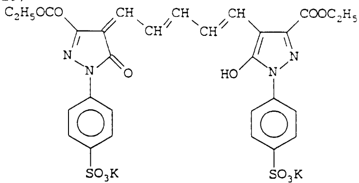
(Cpd - 19)
