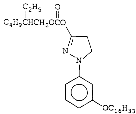
(Cpd - 11)
