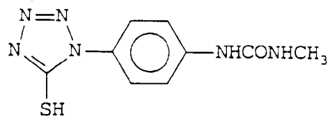
(Cpd - 23)
