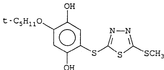
(Cpd - 102)
