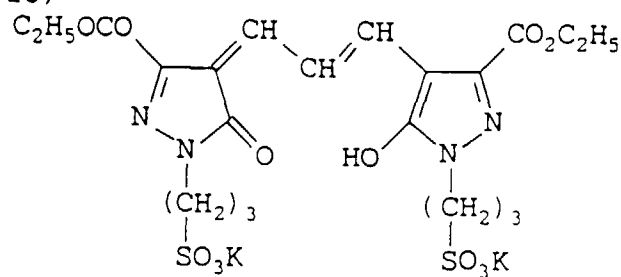
(Cpd - 18)
