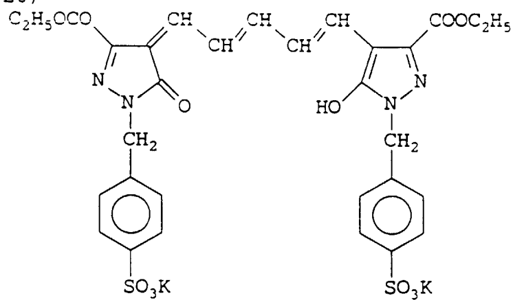
(Cpd - 20)
