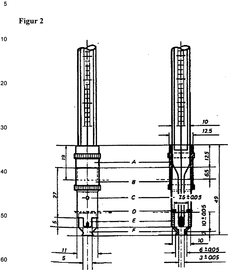
Abb. 2.2.17-1: Apparatur zur Bestimmung des Tropfpunkts Längenangaben in Millimetern
