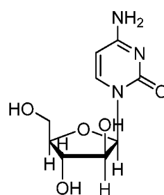
Cytarabine (Ara-C)
