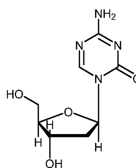
Decitabine
