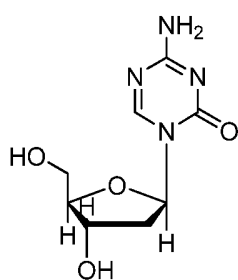
Decitabine
