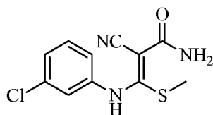
3-((3-chlorophenyl)amino)-2-cyano-3-(methylthio)acrylamide
