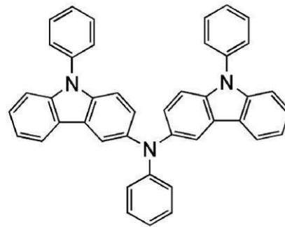
PCzPCA1
