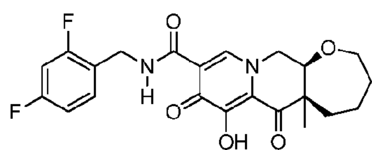
39 (Enantiomer A) 40 (Enantiomer B)
