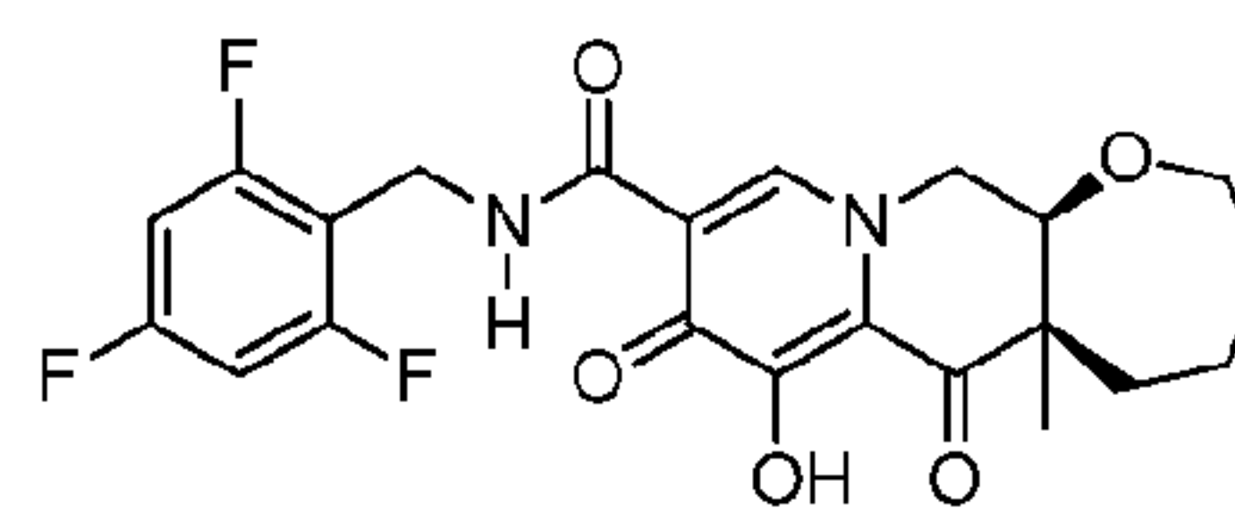
41 (Enantiomer A) 42 (Enantiomer B)
