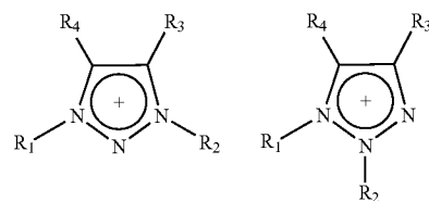
1,2,3-triazolium:
