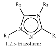
1,2,3-triazolium:
