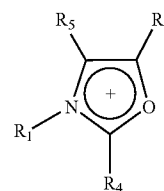
1,2,4-triazolium:
