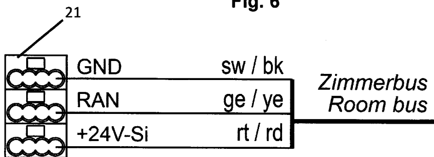
Anschlussprinzip Zimmerbus
