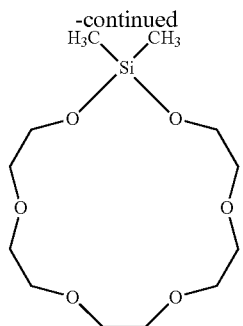
dimethylsila-17-crown-6.
