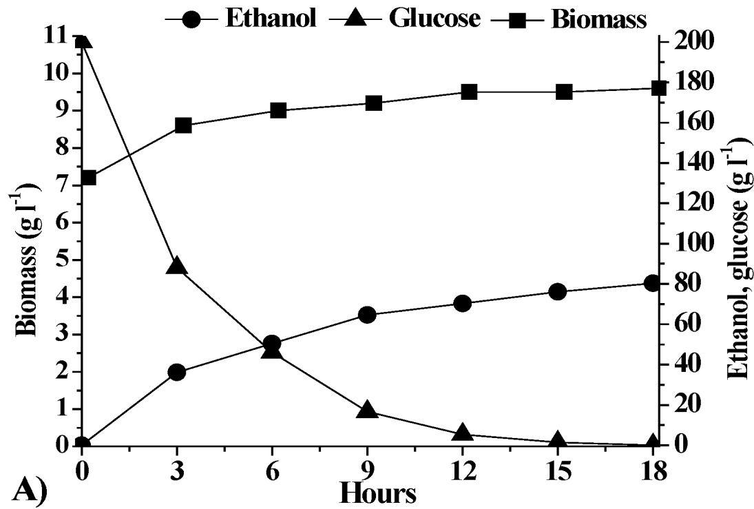
FIG. 1: AS400 fermentation
