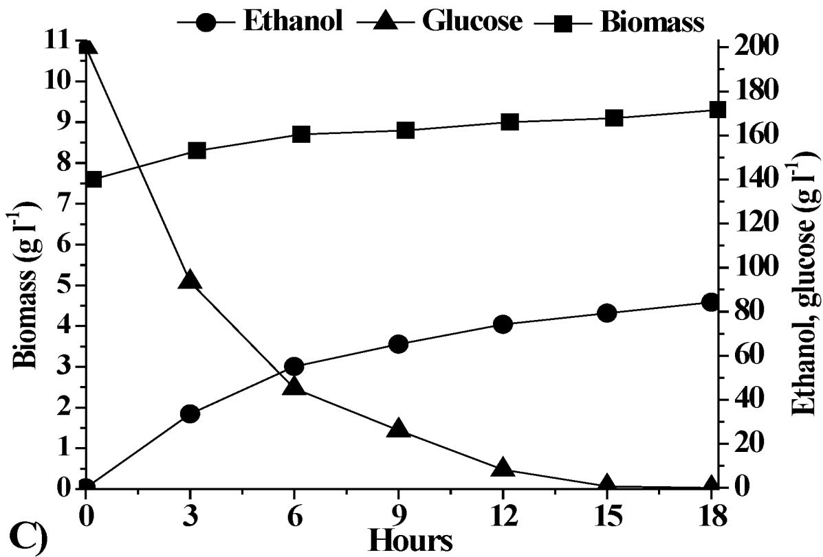
FIG. 3: AS400-543 fermentation
