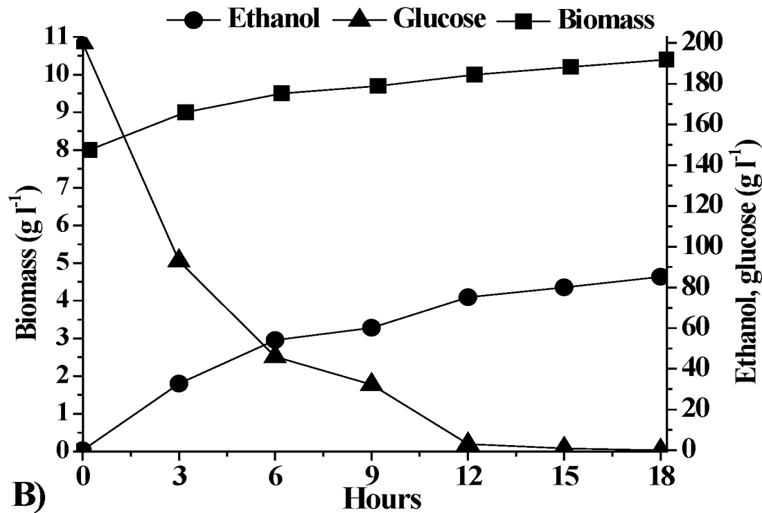
FIG. 2: AS400-567 fermentation
