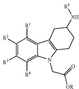
Structure 2a: R 5 ≠ H 2b: R 5 = H
