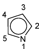
azacyclopentadienyl
