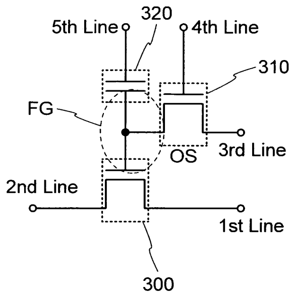
FIG. 8A-1
