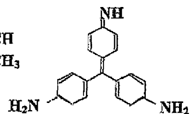
Pararosaniline
