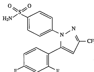
4-[5-(2,4-[Difluoro]phenyl)-3-(trifluoromethyl)-1H-pyrazol-1-yl]benzenesulfonamide
