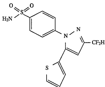
4-[5-(2-Thienyl)-3-(difluoromethyl)-1H-pyrazol-1-yl]-benzenesulfonamide
