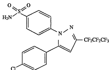
4-[5-(4-Chlorophenyl)-3-(heptafluoropropyl)-1H-pyrazol-1-yl]benzenesulfonamide
