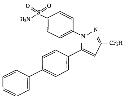
4-[5-(4-Biphenyl)-3-(difluoromethyl)-1H-pyrazol-1-yl]benzenesulfonamide
