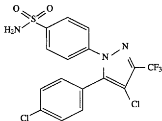
4-[5-(4-Chlorophenyl)-3-(trifluoromethyl)-4-chloro-1H-pyrazol-1-yl]benzenesulfonamide
