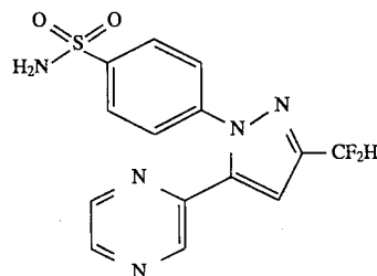
4-[5-(2-Pyrazinyl)-3-(difluoromethyl)-1H-pyrazol-1-yl]benzenesulfonamide
