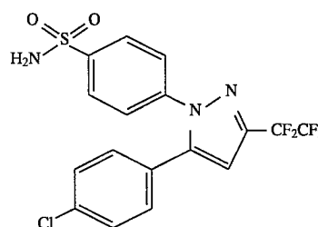
4-[5-(4-Chlorophenyl)-3-(pentafluoroethyl)-1H-pyrazol-1-yl]benzenesulfonamide
