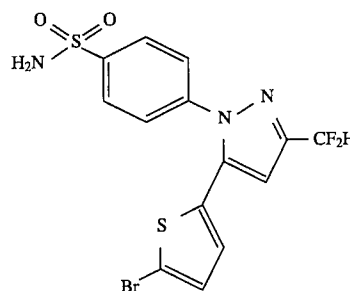
4-[5-(5-Bromo-2-thienyl)-3-(difluoromethyl)-1H-pyrazol-1-yl]benzenesulfonamide
