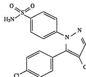
4-[5-(4-Chlorophenyl)-4-chloro-1H-pyrazol-1-yl]benzenesulfonamide
