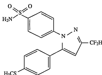
4-[5-(4-[Methylthio]phenyl)-3-(difluoromethyl)-1H-pyrazol-1-yl]benzenesulfonamide
