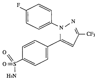
4-[1-(4-Fluorophenyl)-3-(trifluoromethyl)-1H-pyrazol-5-yl]benzenesulfonamide
