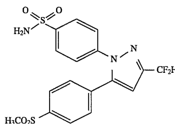
4-[5-(4-[Methylsulfonyl]phenyl)-3-(difluoromethyl)-1H-pyrazol-1-yl]benzenesulfonamide
