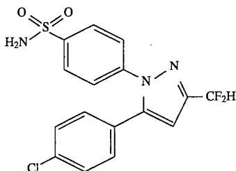
4-[5-(4-Chlorophenyl)-3-(difluoromethyl)-1H-pyrazol-1-yl]benzenesulfonamide
