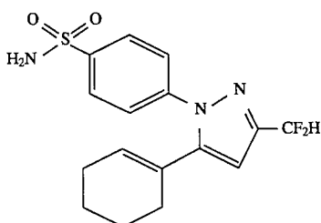
4-[5-(1-Cyclohexenyl)-3-(difluoromethyl)-1H-pyrazol-1-yl]benzenesulfonamide
