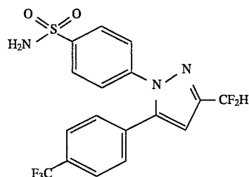
4-[5-(4-[Trifluoromethyl]phenyl)-3-(difluoromethyl)-1H-pyrazol-1-yl]benzenesulfonamide
