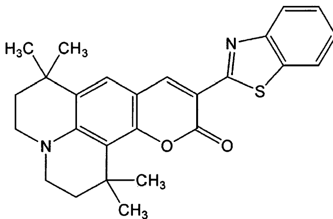
C545T
