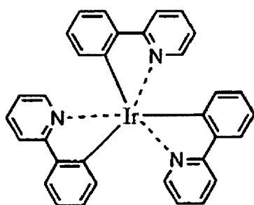
Ir(ppy) 3
