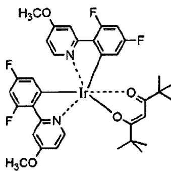
(F_2ppy)_2Ir(tmd)
