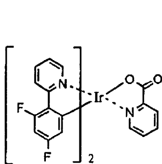
F_2Irpic
