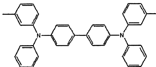
TPD
