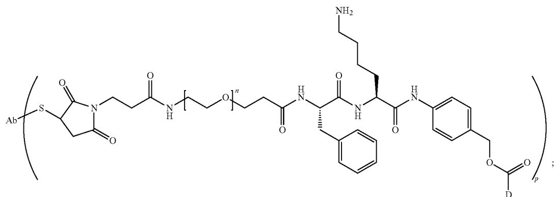
Phe-homoLys-PAB-Ab
