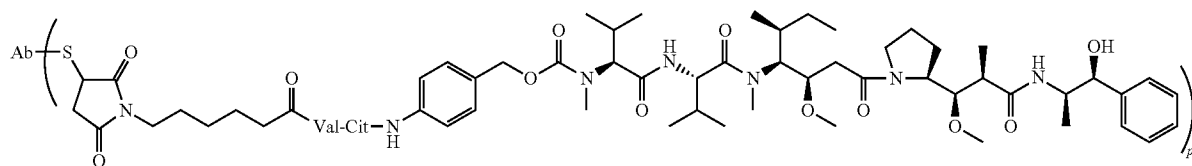
Ab-MC-vc-PAB-MMAE
