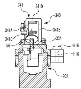
(B) T-T断面図
