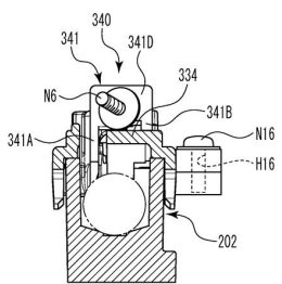
(D) U-U断面図
