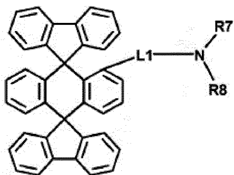
[Formule Chimique 1-2]
