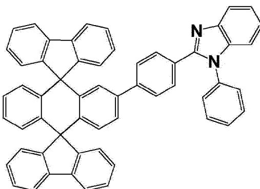
[ET 2]
