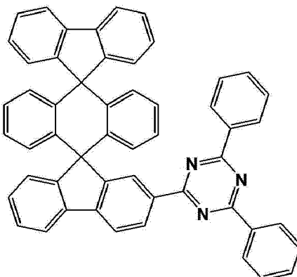
[RH 3]
