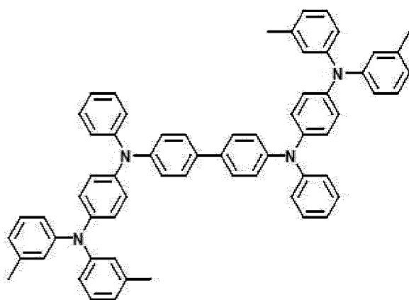
[DNTPD]
