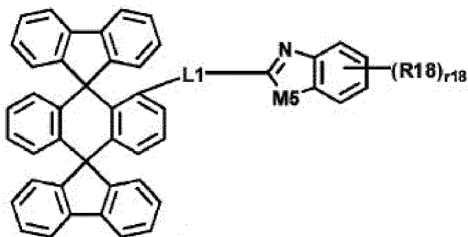
[Formule Chimique 1-6]
