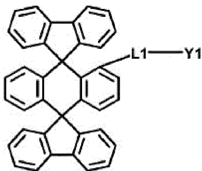
[Formule Chimique 1-1]
