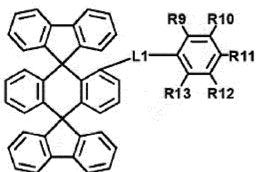
[Formule Chimique 1-3]
