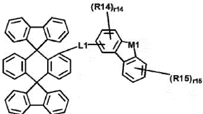
[Formule Chimique 1-4]
