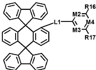
[Chemische Formel 1-5]
