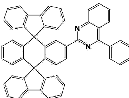
[RH 2]
