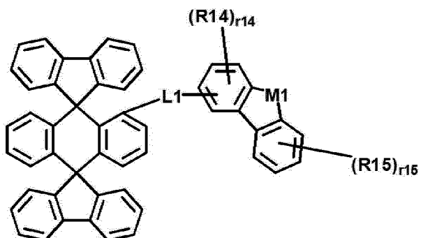
[Chemische Formel 1-5]
