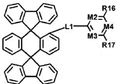
[Formule Chimique 1-5]
