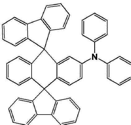
[EB 2]
