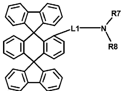
[Chemische Formel 1-3]
