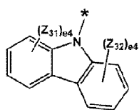
化学式 5-20
