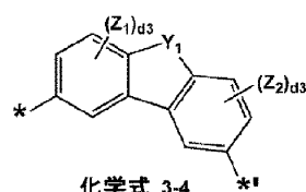
化学式 3-4
