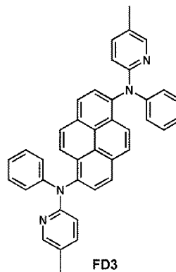
FD3
