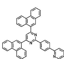
ET22
