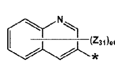
化学式 5-40
