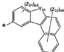
化学式 5-17
