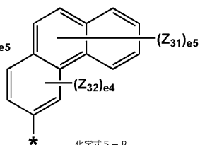
化学式 5-8
