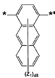
化学式 3-36
