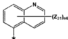
化学式 5-36
