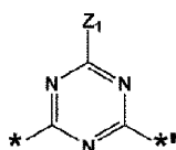
化学式 3-24
