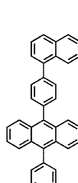
ET21
