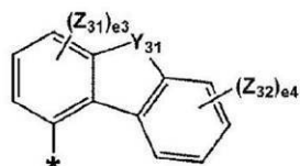
化学式 5-16
