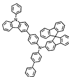
HT8
