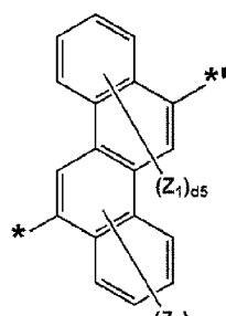
化学式 3-41
