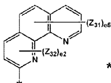
化学式 5-21
