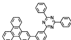
H52
