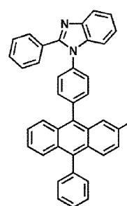
ET15
