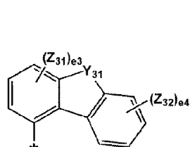
化学式 5-16
