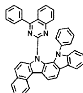
H46
