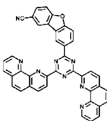
137
