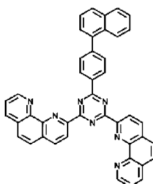
140
