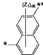
化学式 3-33
