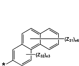
化学式 5-9
