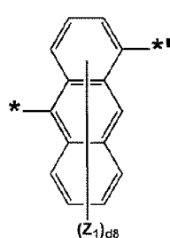
化学式 3-37
