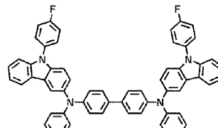
HT30
