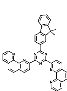
133
