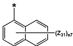
化学式 5-3
