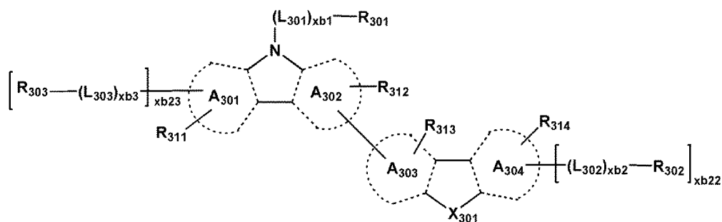
301-2
