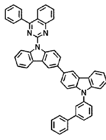
H41
