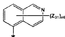
化学式 5-35
