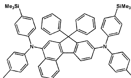
FD21
