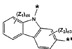
化学式 3-32
