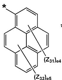
化学式 5-10
