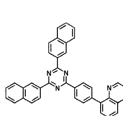
ET27
