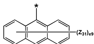
化学式 5-4
