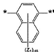
化学式 3-6
