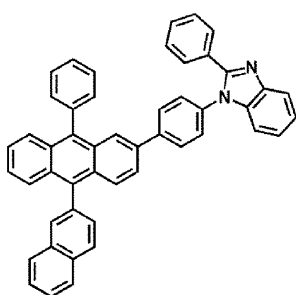
ET13
