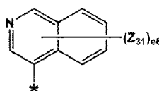
化学式 5-38
