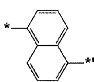
化学式 4-8
