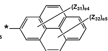
化学式 5-12
