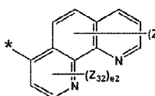
化学式 5-23
