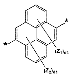
化学式 3-39
