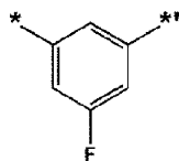
化学式 4-6
