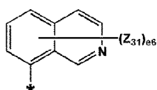
化学式 5-34
