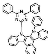
H45
