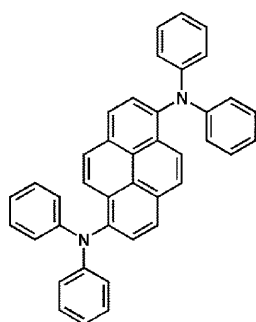
FD1
