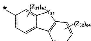
化学式 5-14
