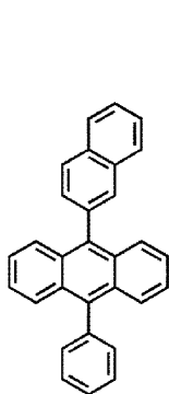
ET19
