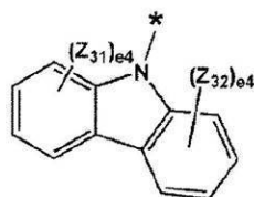
化学式 5-20
