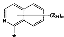
化学式 5-39
