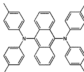
FD16
