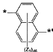
化学式 3-7
