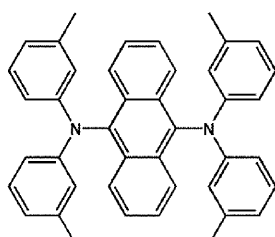
FD15
