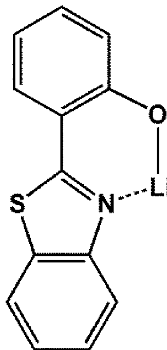
ET-D2
