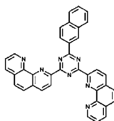
139
