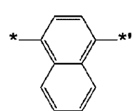
化学式 4-7
