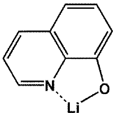
ET-D1
