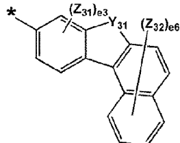
化学式 5-18
