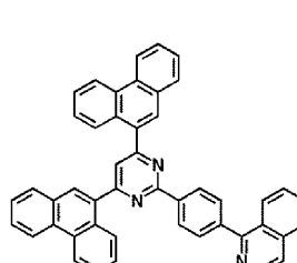
ET24
