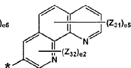
化学式 5-22
