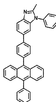
ET18
