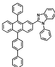
ET14
