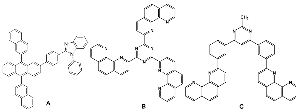
【化 1 0 7】
