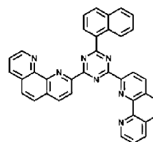
138
