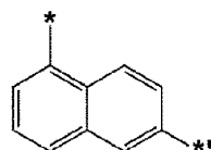
化学式 4-11
