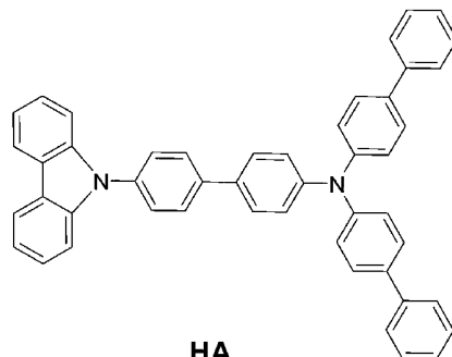
HA
