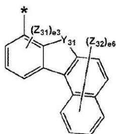
化学式 5-19
