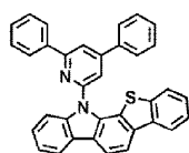
H44
