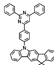
H43
