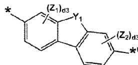
化学式 3-3
