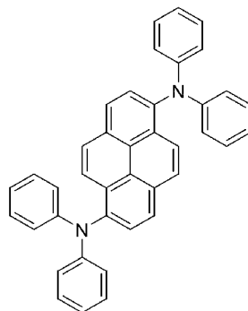
TPD
