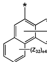
化学式 5-7
