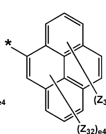
化学式 5-11
