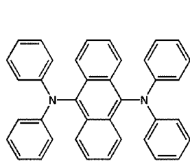
FD14
