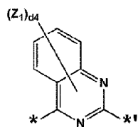
化学式 3-28
