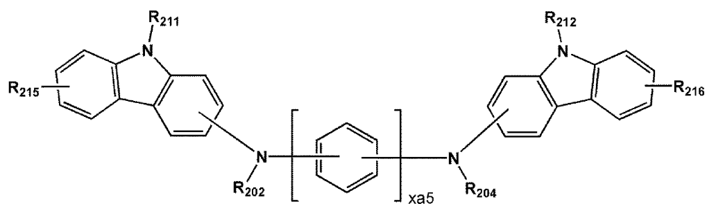
202A
