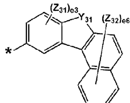
化学式 5-17
