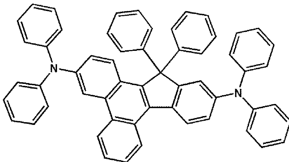
FD22
