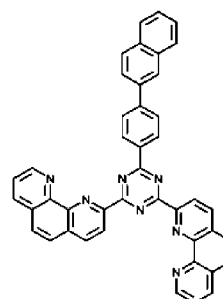
141
