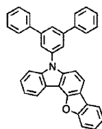
H42
