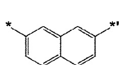
化学式 4-10
