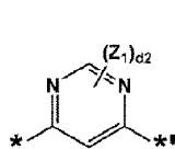
化学式 3-23
