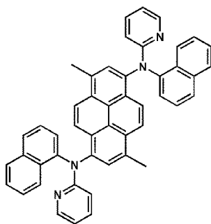
FD2
