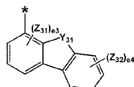
化学式 5-15
