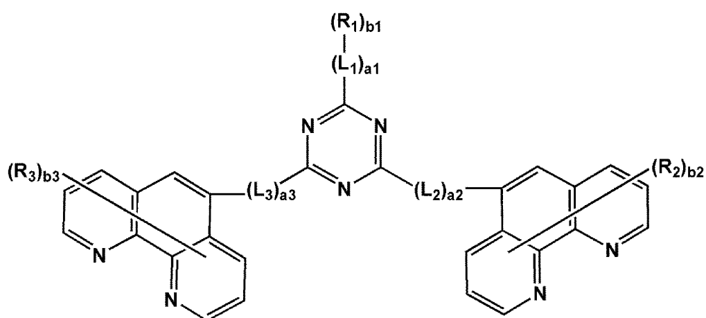
1 - 4
