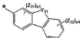
化学式 5-14
