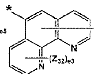
化学式 5-24
