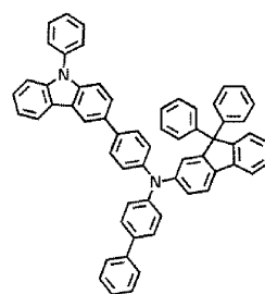
HT6
