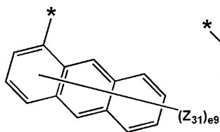
化学式 5-5
