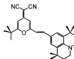
DCJTB
