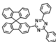
H53
