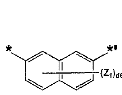
化学式 3-34
