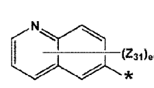
化学式 5-41
