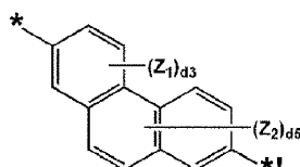
化学式 3-25
