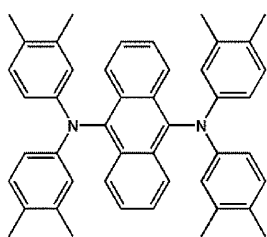
FD17
