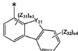
化学式 5-15
