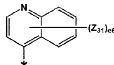
化学式 5-37
