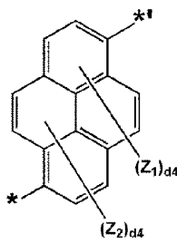
化学式 3-38
