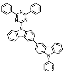
H40
