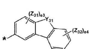
化学式 5-13
