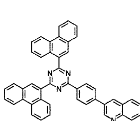
ET25
