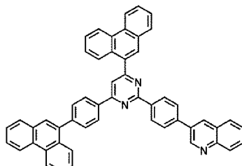
ET23
