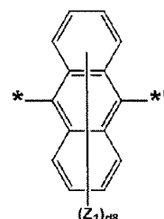
化学式 3-8
