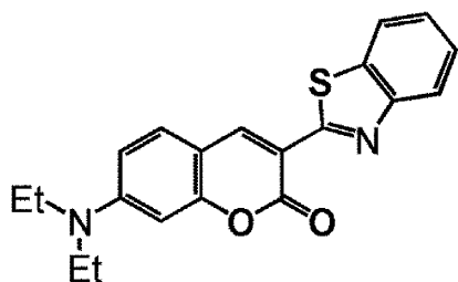
Coumarin 6
