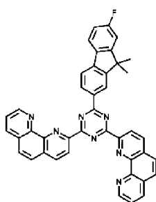
134
