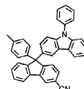
H54
