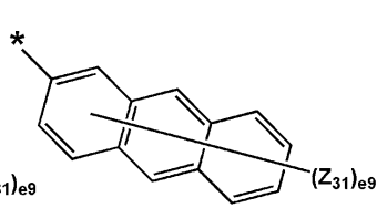
化学式 5-6
