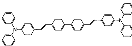
DPAVB
