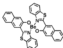
H55
