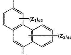
化学式 3-35
