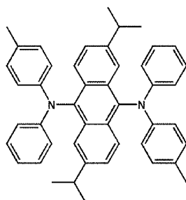
FD18
