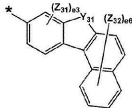
化学式 5-18
