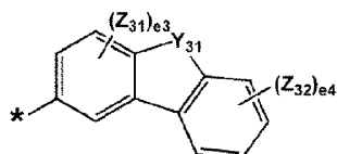
化学式 5-13
