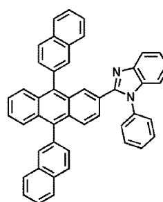
ET12
