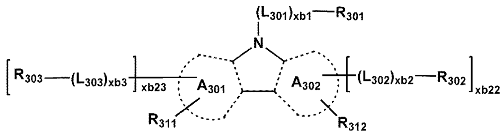
301-1
