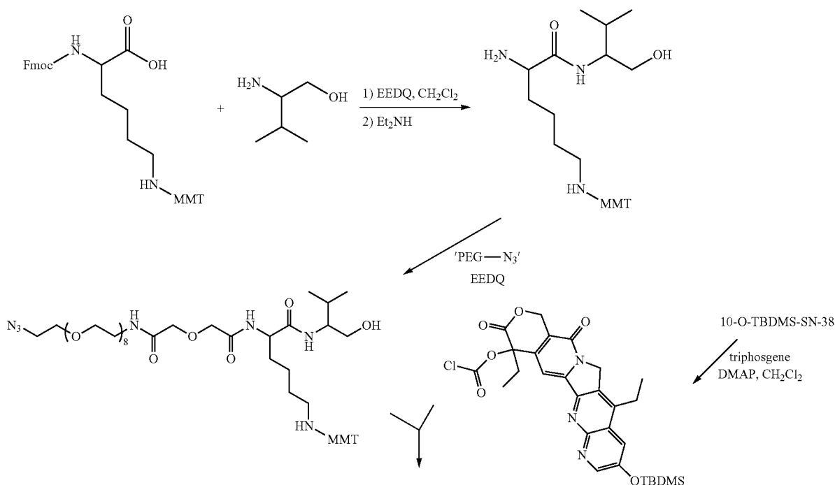
Scheme-2
