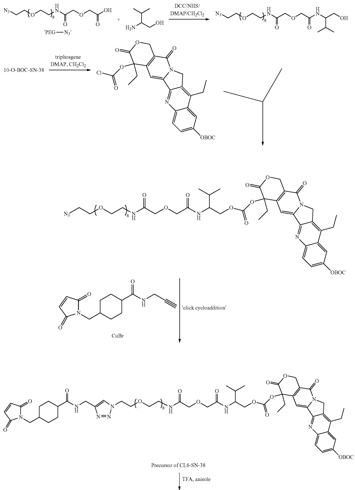
Scheme-1
