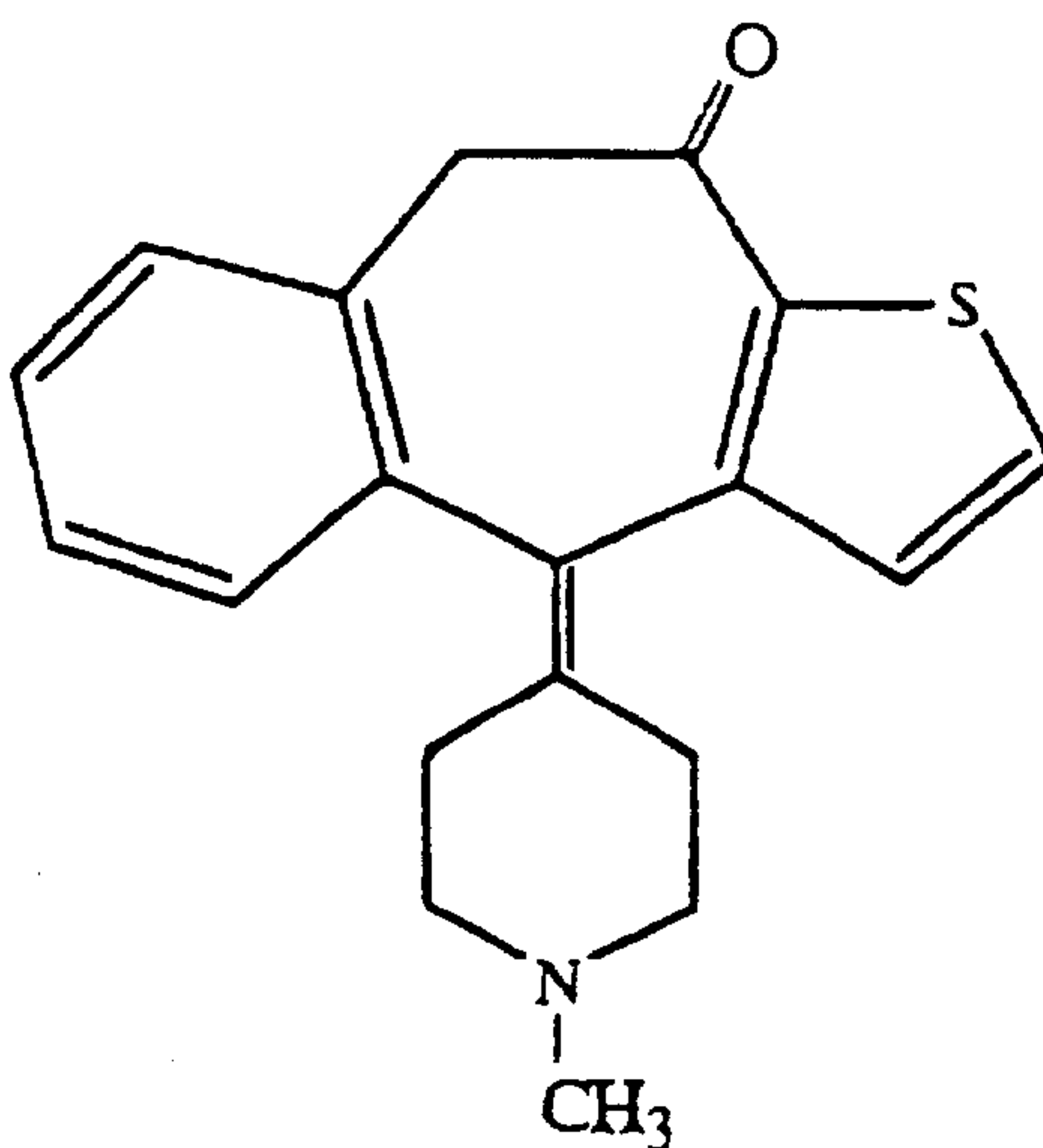
KETOTIFEN
