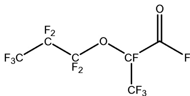
Compound D1
