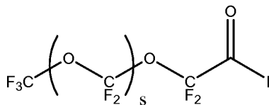
Compound D2
