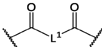
Formula L-1
