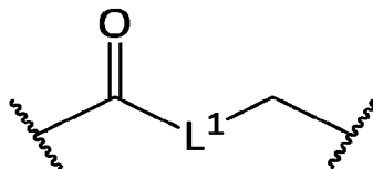
Formula L-1
