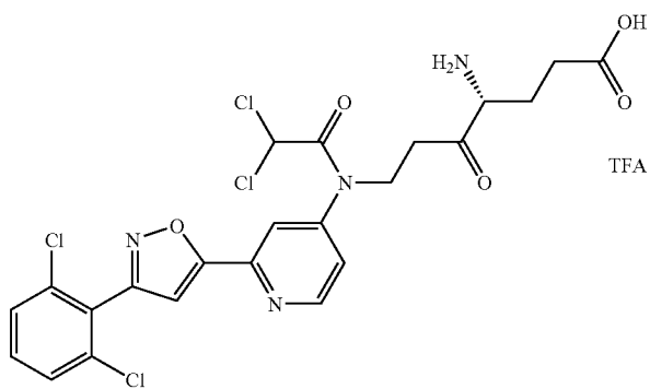
Cpd. No. 4
