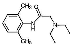
Lidocaine (71)
