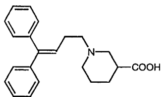
SKF 89976-A (53)
