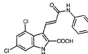
GV150526A ( 14d )
