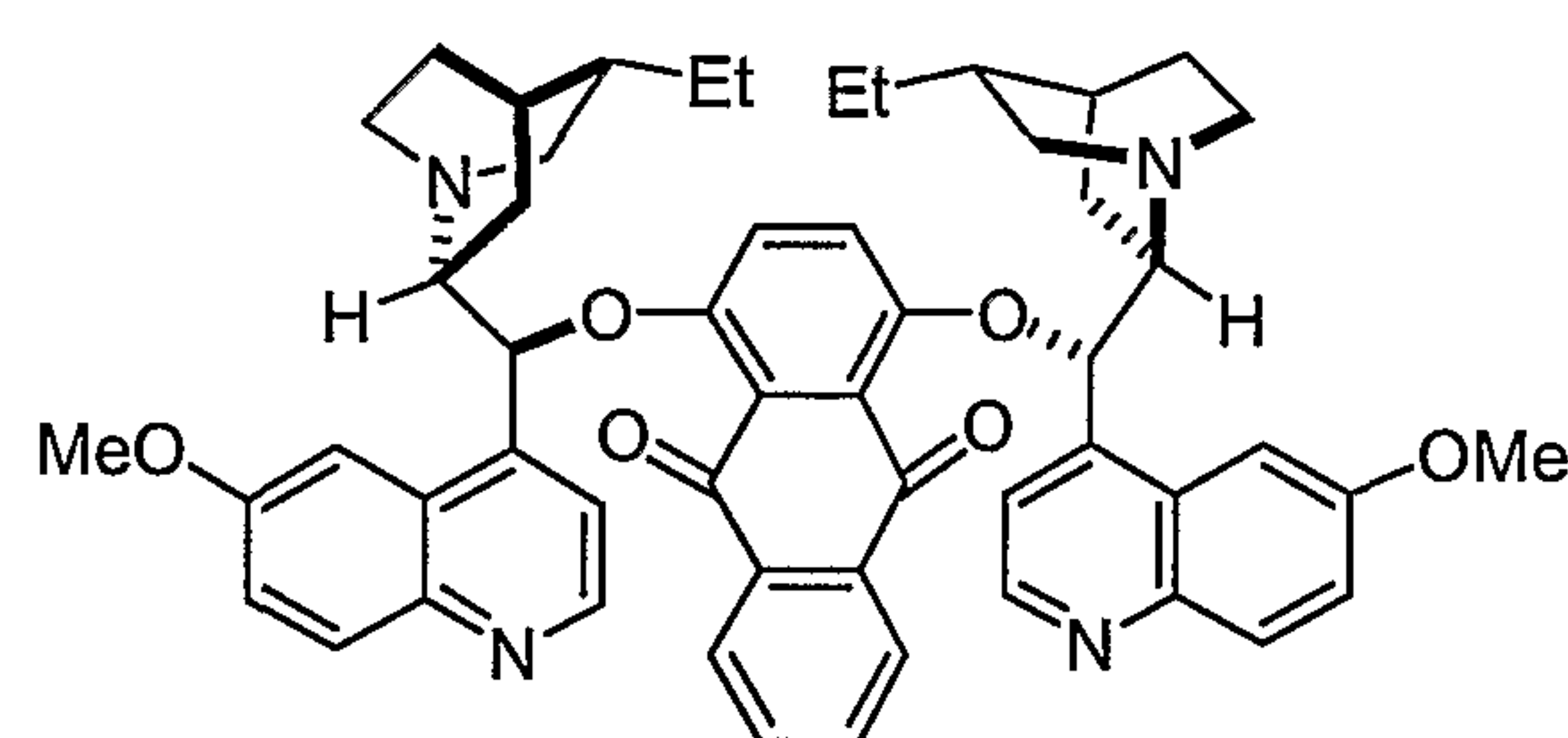
(DHQD) 2 AQN
