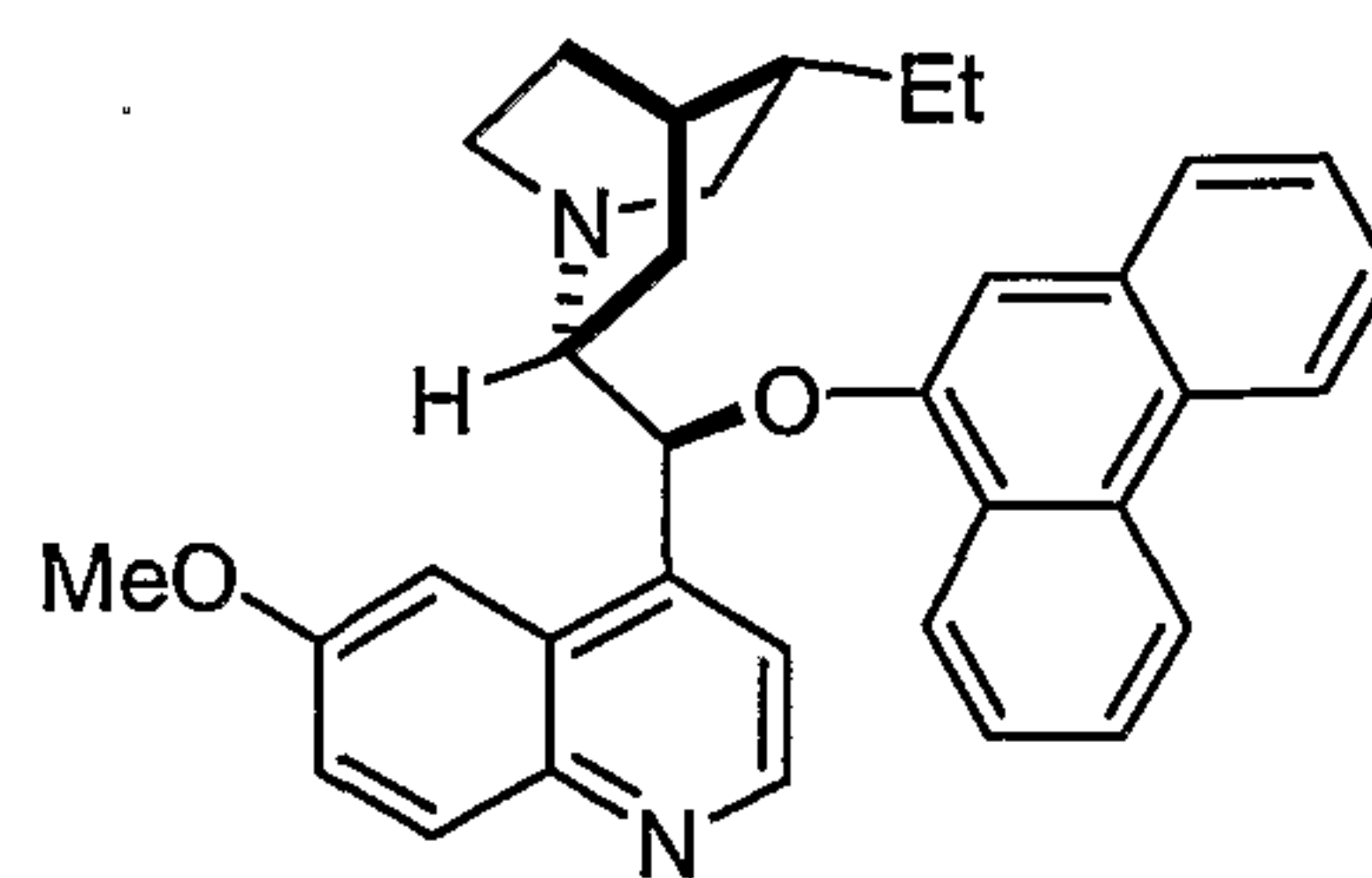
DHQD-PHN
