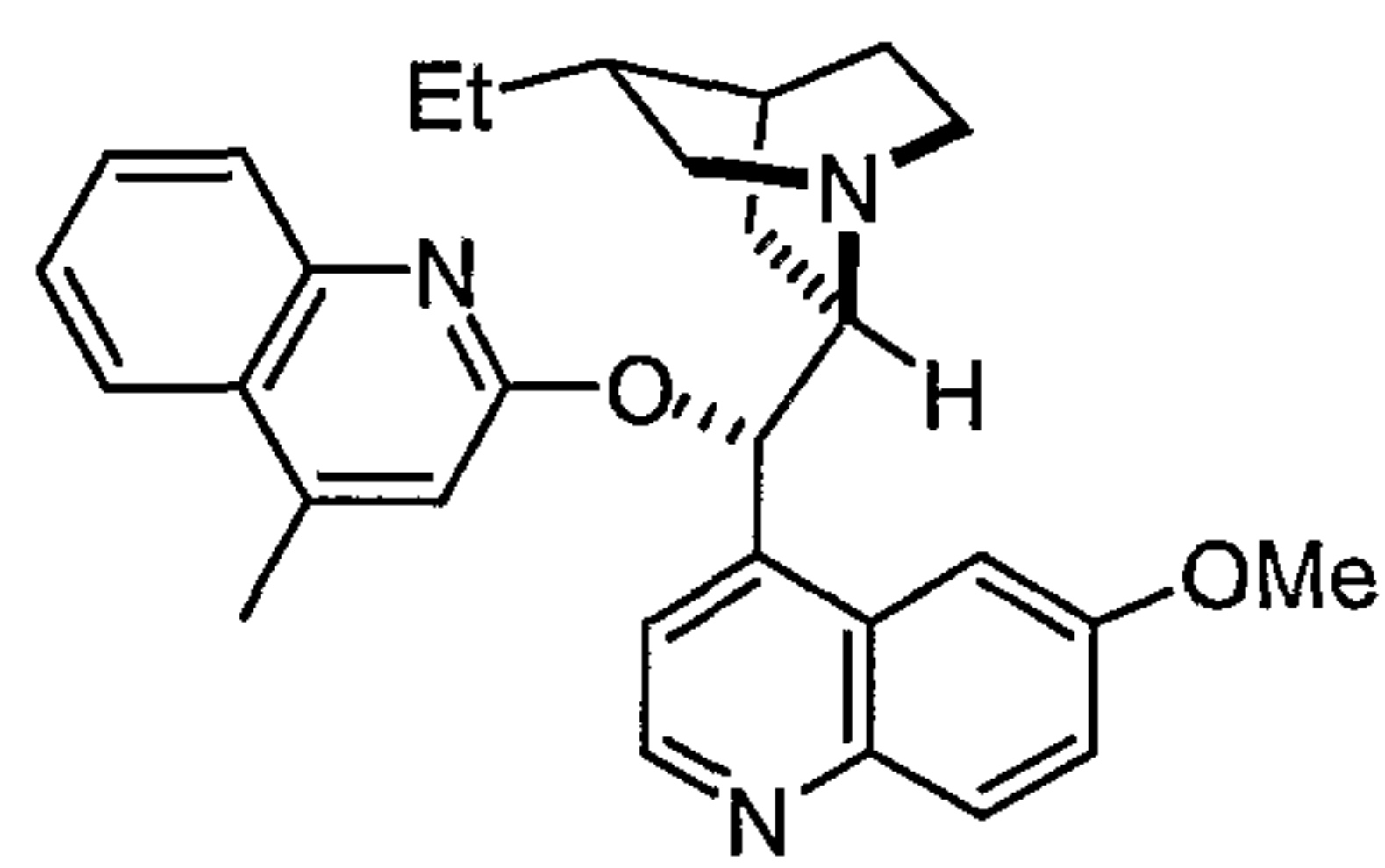
DHQD-MEQ
