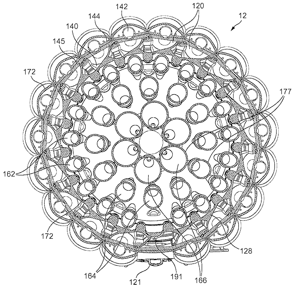
B - B FIG. 6(b)
