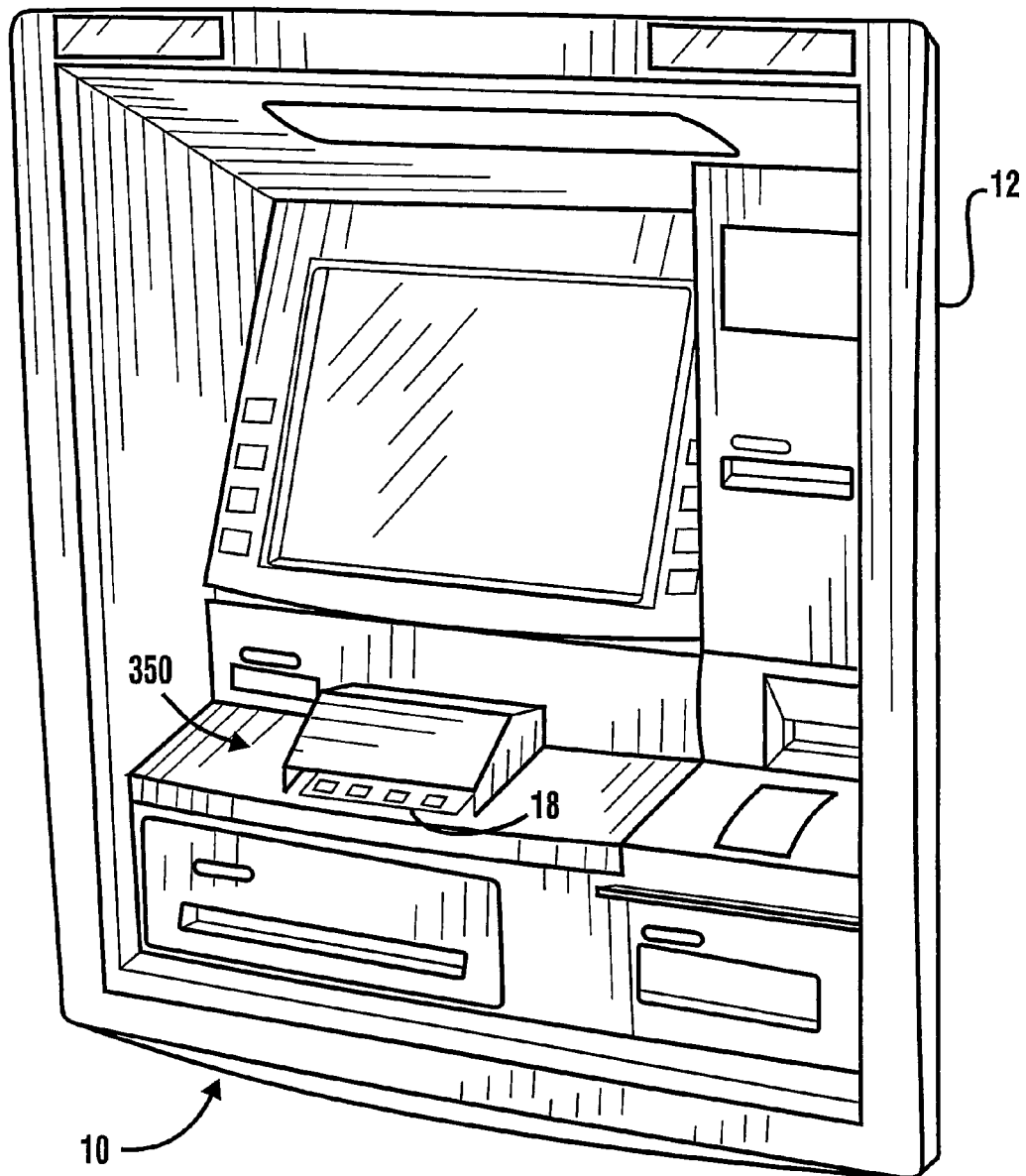
FIG. 28
