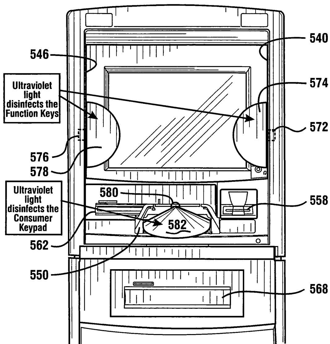
Fig. 49
