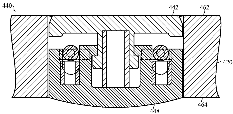
SECTION C-C FIG. 10A
