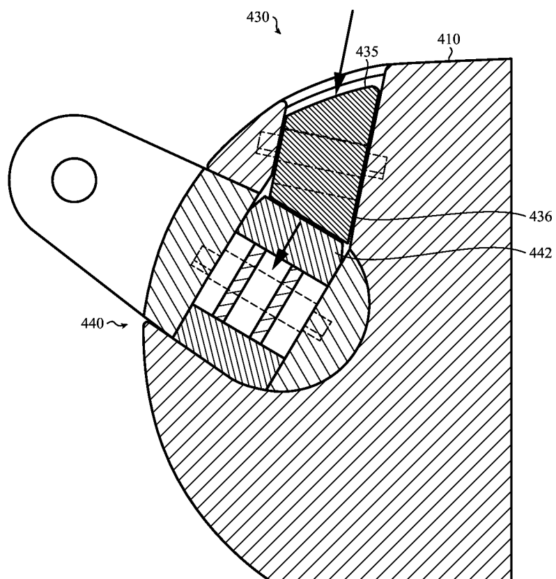
SECTION B-B FIG. 13B
