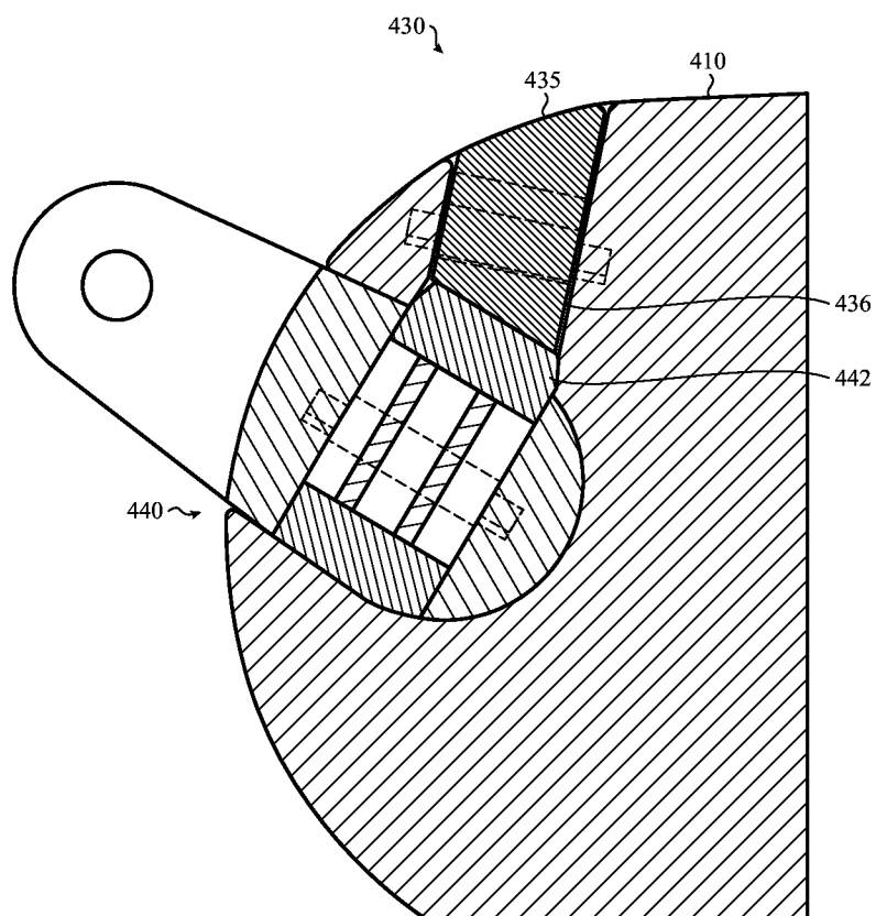
SECTION B-B FIG. 13A
