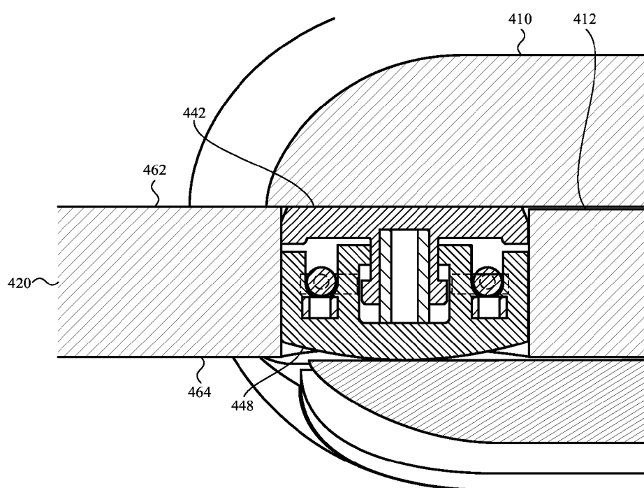
SECTION A-A FIG. 12B
