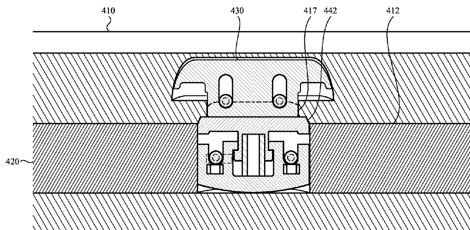
SECTION A-A FIG. 12C
