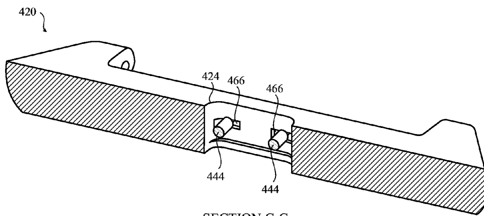
SECTION C-C FIG. 9A
