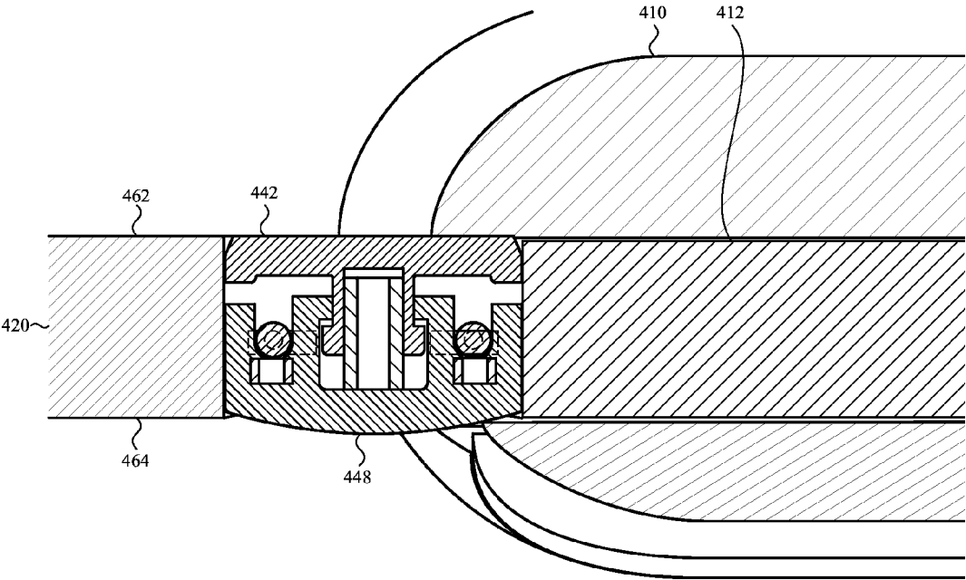
SECTION A-A FIG. 12A
