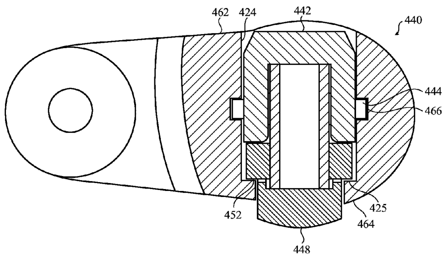
SECTION D-D FIG. 8B
