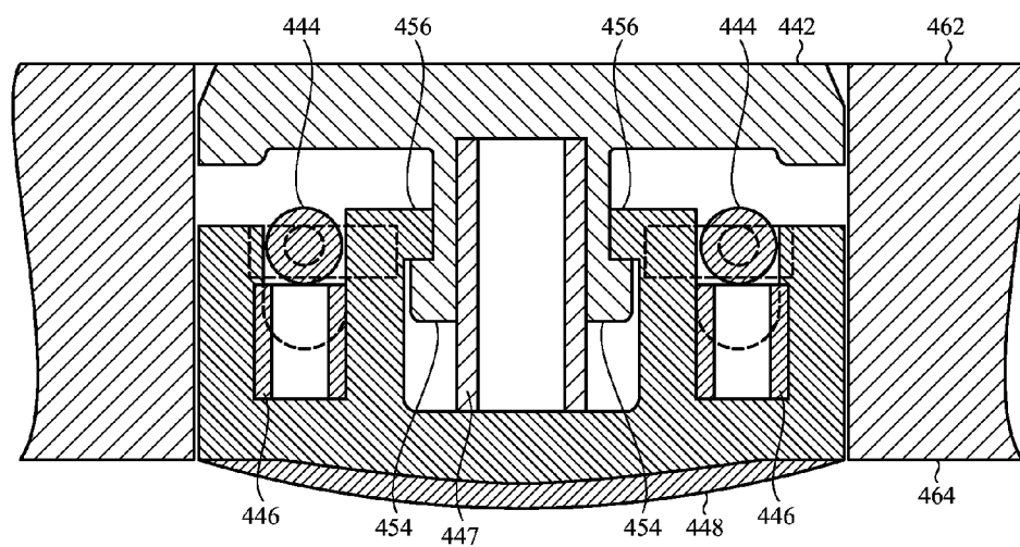
SECTION C-C FIG. 8A
