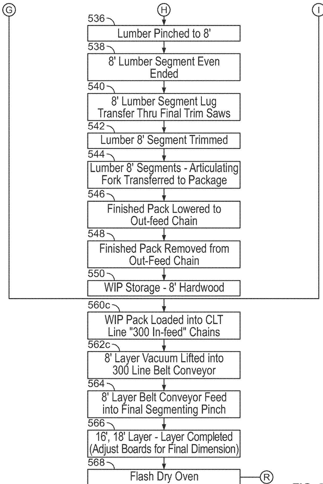
FIG. 5A-6
