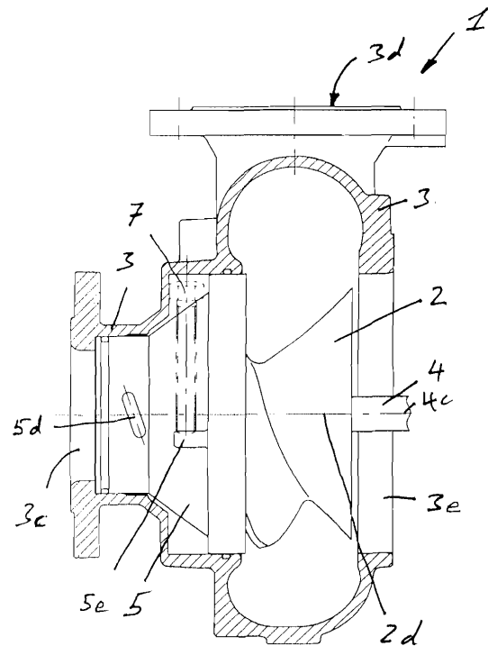
Fig. 3(A-A)
