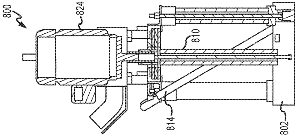
SECTION G-G FIG. 8T
